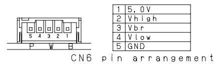
Fig. 5 LQ281L1LW11 MODULE OUTLINE 2/2
