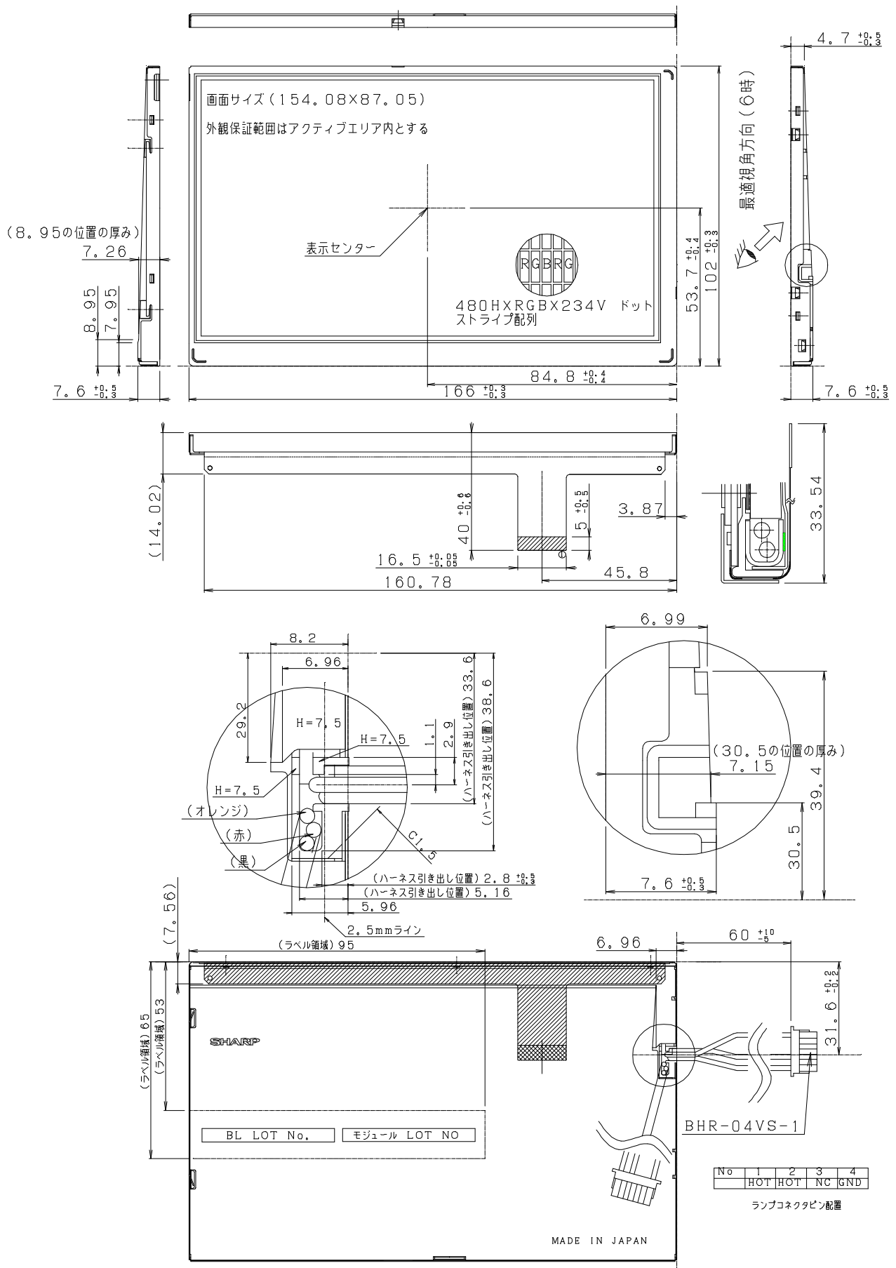
図1 モジュール外形図
