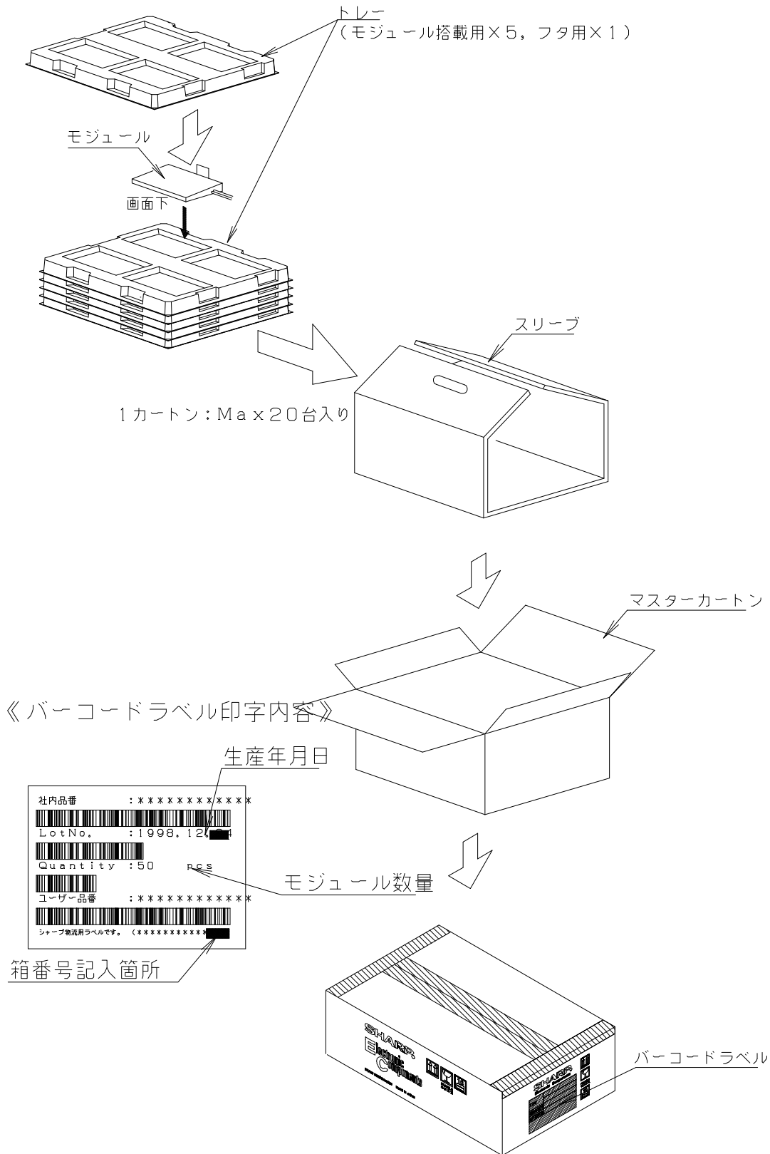
図5. 包装形態図
