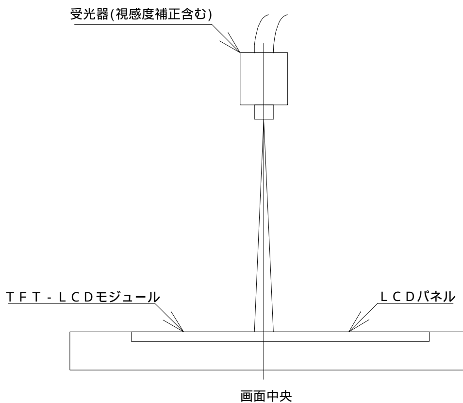
光学的特性測定方法
