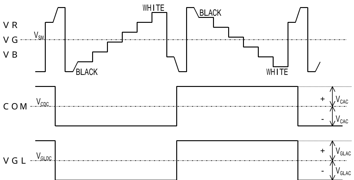
図4 入力信号タイミング図
